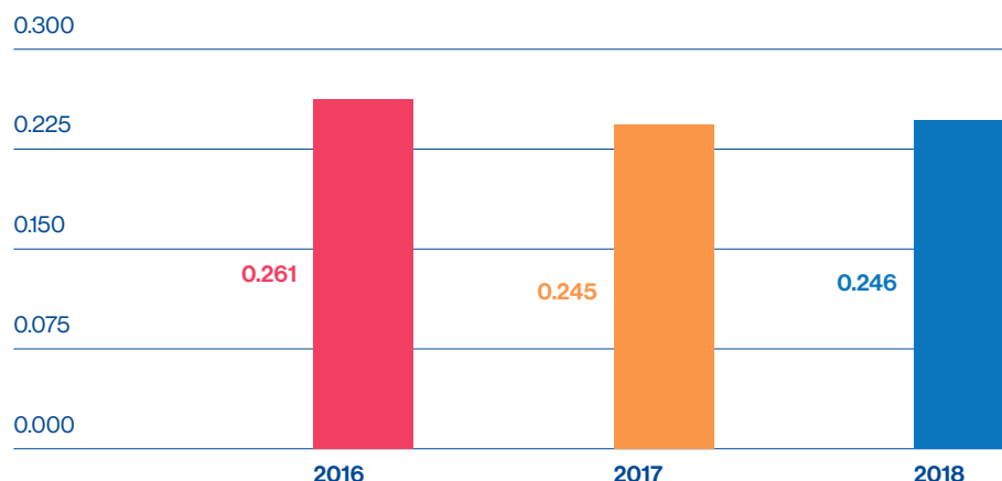
Figura 7 Consumo di energia elettrica per ton di vetro fuso 2016-2018 (16 aziende)
