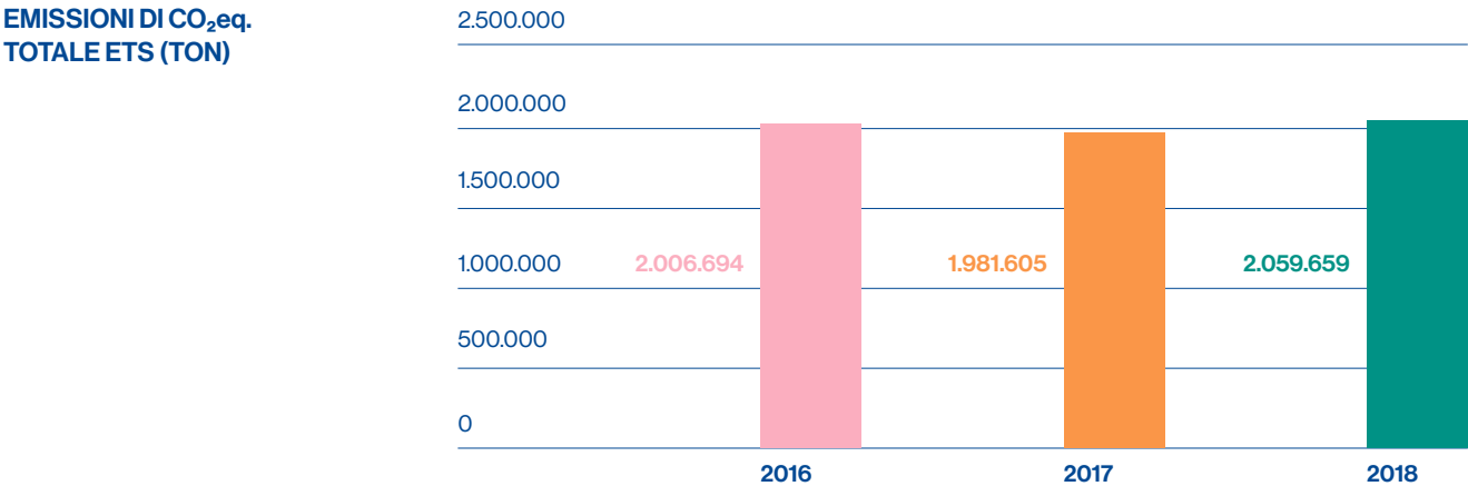
Figura 12 Emissioni di CO 2 eq totale ETS 2016-2018 (16 aziende)
