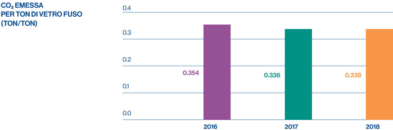
Figura 11 Emissioni di CO 2 da forno per ton di vetro fuso 2016-2018 (15 aziende)
