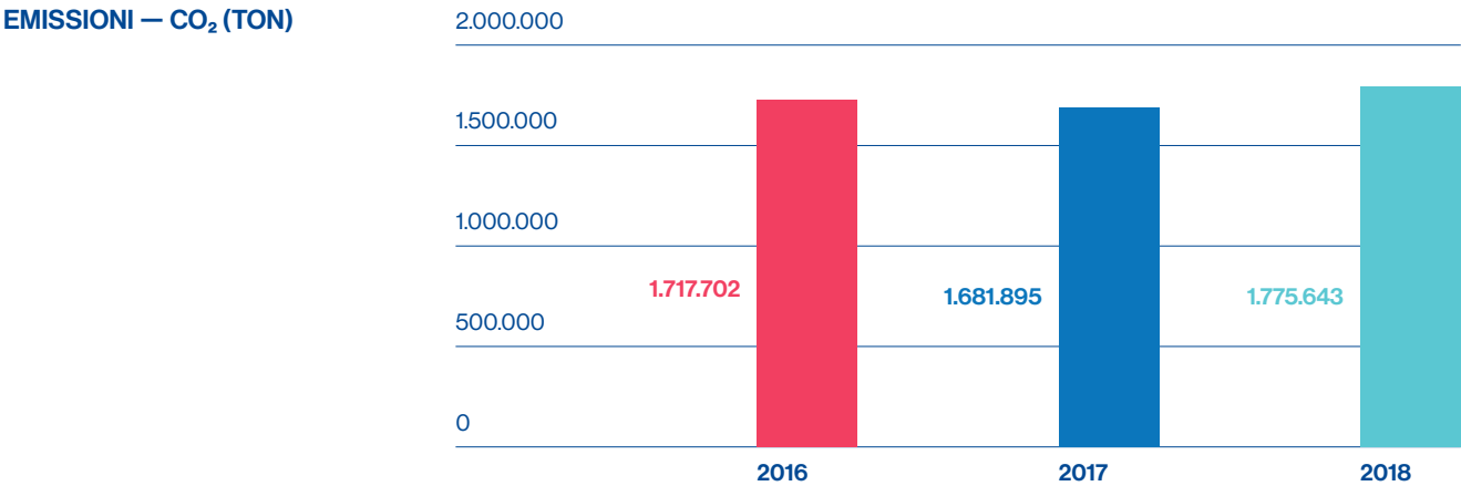
Figura 10 Emissioni di CO 2 da forno 2016-2018 (15 aziende)
