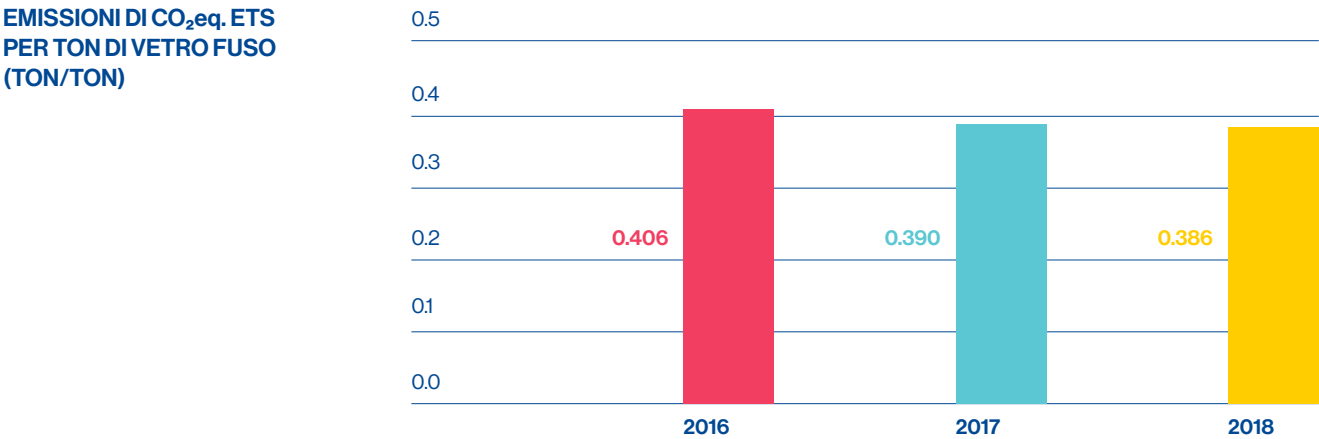
Figura 13 Emissioni di CO 2 eq. ETS per ton di vetro fuso 2016-2018 (16 aziende)
